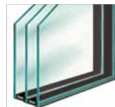
Aufpreis Wärmeschutzglas, 3-fach Therm Ultra 0.7 WE Glasaufbau 4-12-4-12-4 mm U_g: 0,7 \text{ W/m}^2 \text{ K} R_w: 35 \text{ dB}
