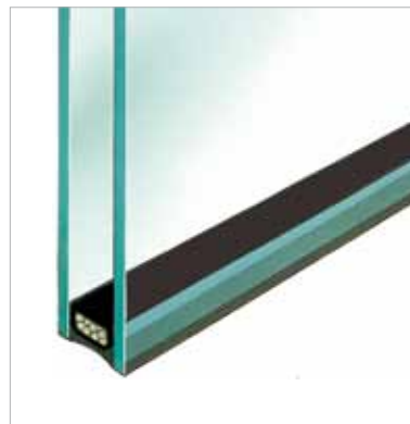
Corona S Wärmeschutzglas Therm Ultra 1.1 WE Glasaufbau 4-16-4 mm U_g: 1,1 \text{ W/m}^2 \text{ K} R_w: 32 \text{ dB}
