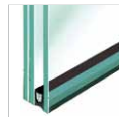
Aufpreis Einbruchhemmendes Glas Therm Ultra 1.1 WE A3 Glasaufbau A3 (10)-16-4 mm U_g: 1,1 \text{ W/m}^2 \text{ K} R_w: 38 \text{ dB}
