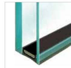
Aufpreis Schallschutzglas Phon Ultra 38 WE Glasaufbau 10-16-4 mm U_g: 1,1 \text{ W/m}^2 \text{ K} R_w: 38 \text{ dB}
